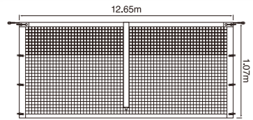
●全天候式上部ダブル硬式テニスネットの規格サイズ
